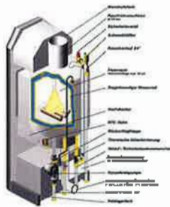
Schnittansicht GD 8 RLU
